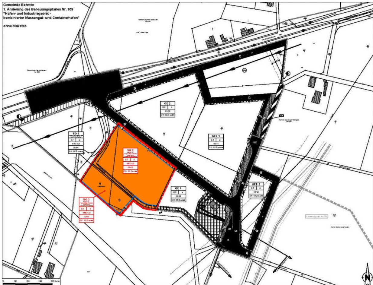
Abbildung 8: 1. Änderung des Bebauungsplan Nr. 109 „Hafen- und Industriegebiet – kombinierter Massengut- und Containerhafen“, ohne Maßstabsangabe
