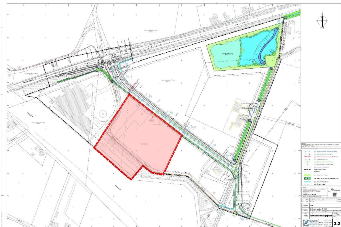
Abbildung 15:: Entwässerungsplan B-Plan Nr. 99 und B-Plan Nr. 109 (IST 2017), verändert: rote Fläche = Bereich der 1. Änderung des B-Plan Nr. 109)
