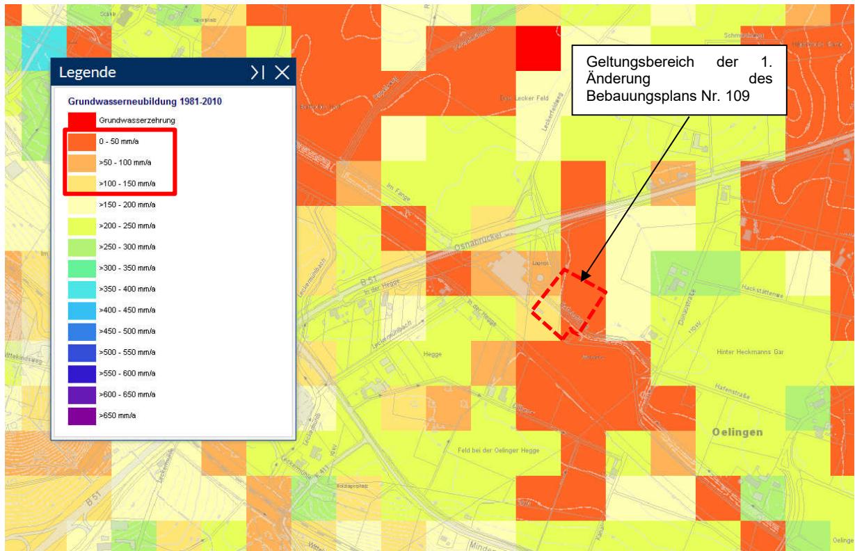
Abbildung 13: Grundwasserneubildung, ohne Maßstabsangabe (LBEG 2022)
